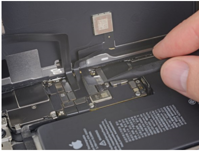
iPhone 11 Pro Substituição Módulo de carga
