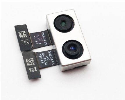
Câmara Traseira de 12Mpx 12Mpx para Xiaomi Mi A1
