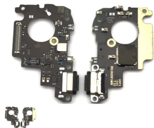
Flex ou módulo de carga para Xiaomi Mi 9 M1902F1G
