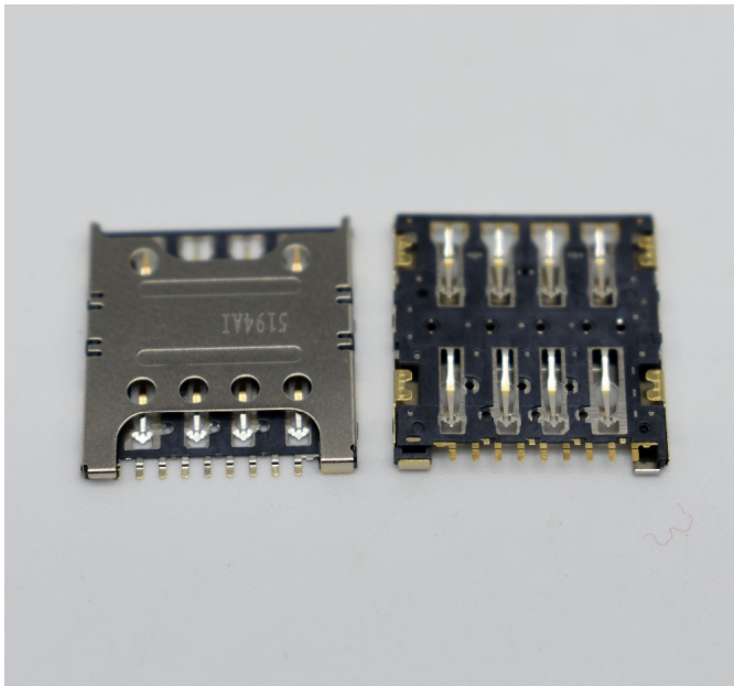
Leitor de cartões Sim micro para Huawei G750
