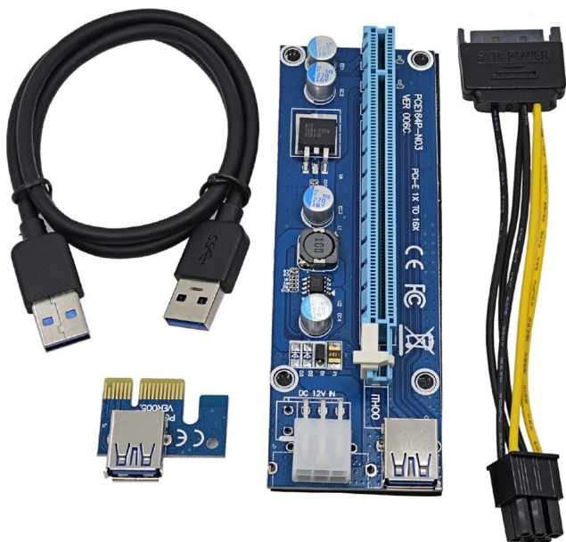
Riser para PCI-E 1X para PCI-E 16X ver.006C
