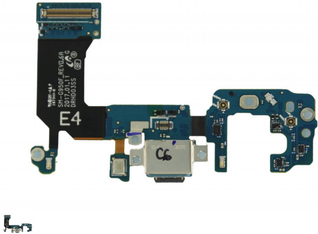
Samsung S8 Substituição da Placa de Carga
