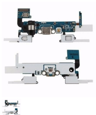
Flex conector de carga, micrófone para Samsung Galaxy A500F
