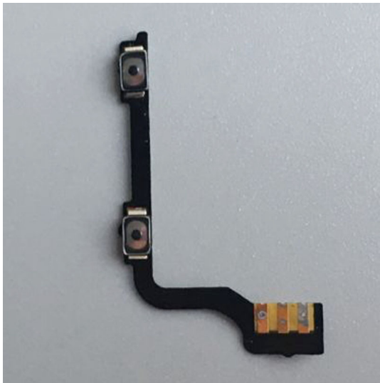
Flex de botões de volume laterais para Oneplus One
