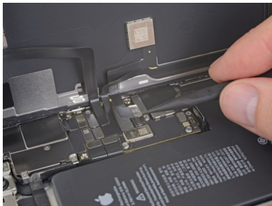
iPhone 11 Substituição Módulo de carga
