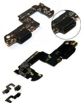
Placa auxiliar com conector USB Tipo C para Honor 9
