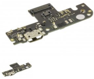
Conector Micro USB para Xiaomi Redmi Note 5A
